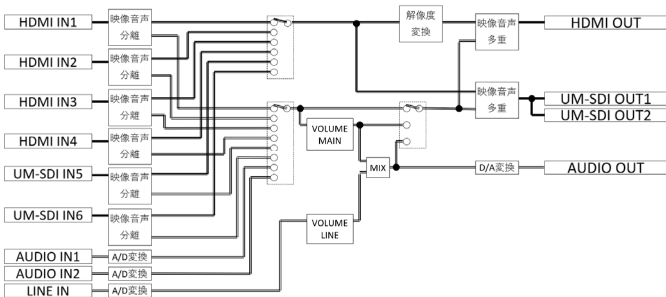
・映像音声スイッチブロック図(6入力1系統出力)
