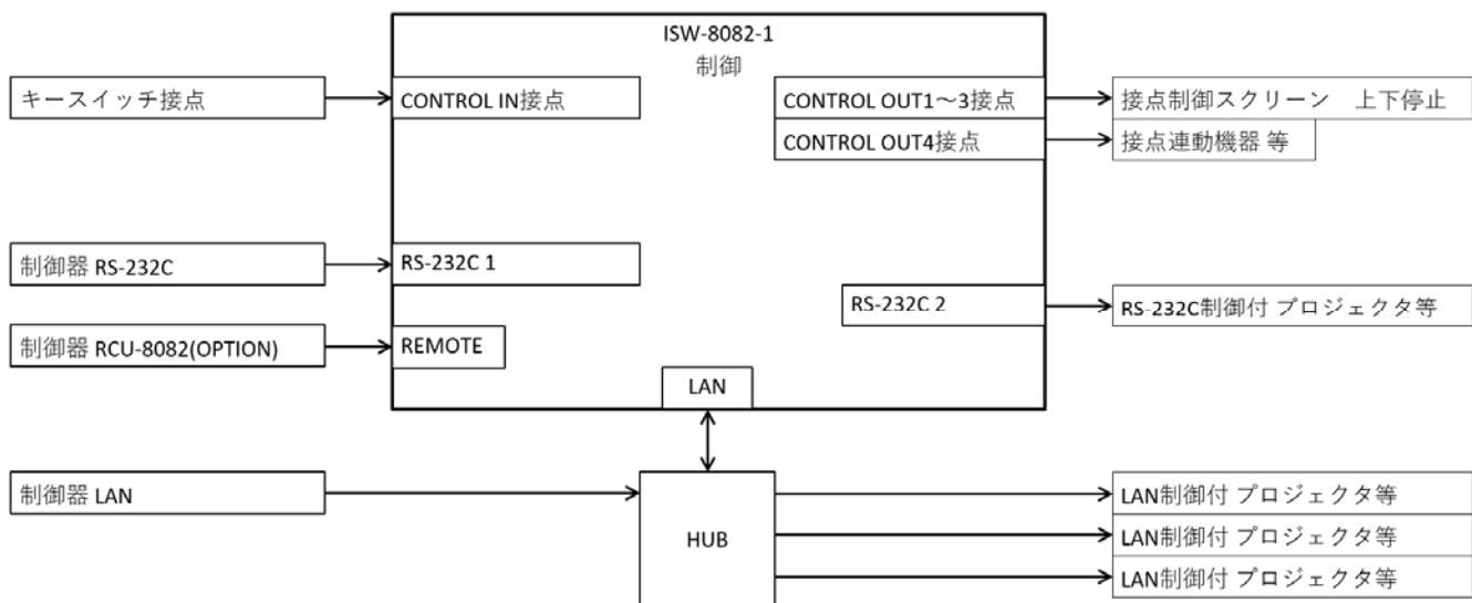
・制御ブロック図
