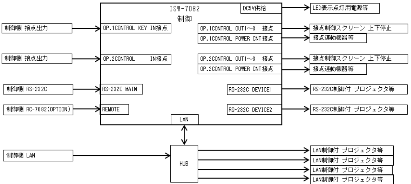
・制御ブロック図
