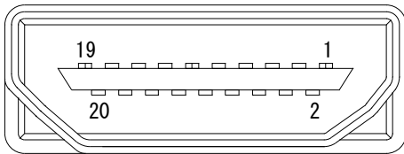
入出力共通 コネクタ:HDMI TYPE A
