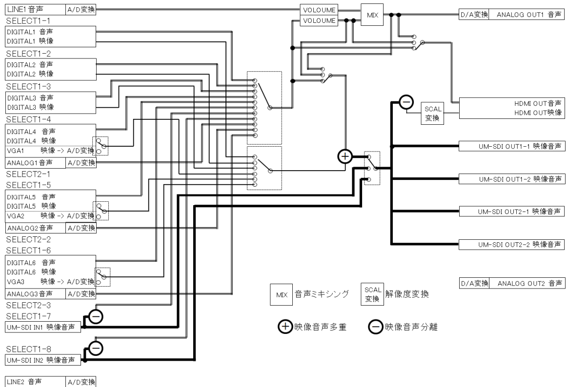
・映像音声スイッチブロック図(11入力1出力モード)
